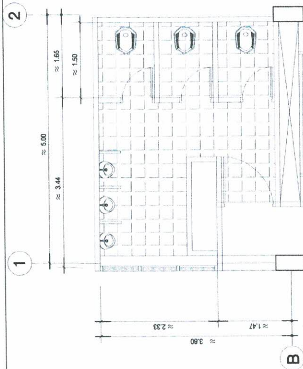
แปลนห้องน้ำชาย ชั้นที่ 1,2,3 ด้านซ้าย (ก่อนการปรับปรุง)
